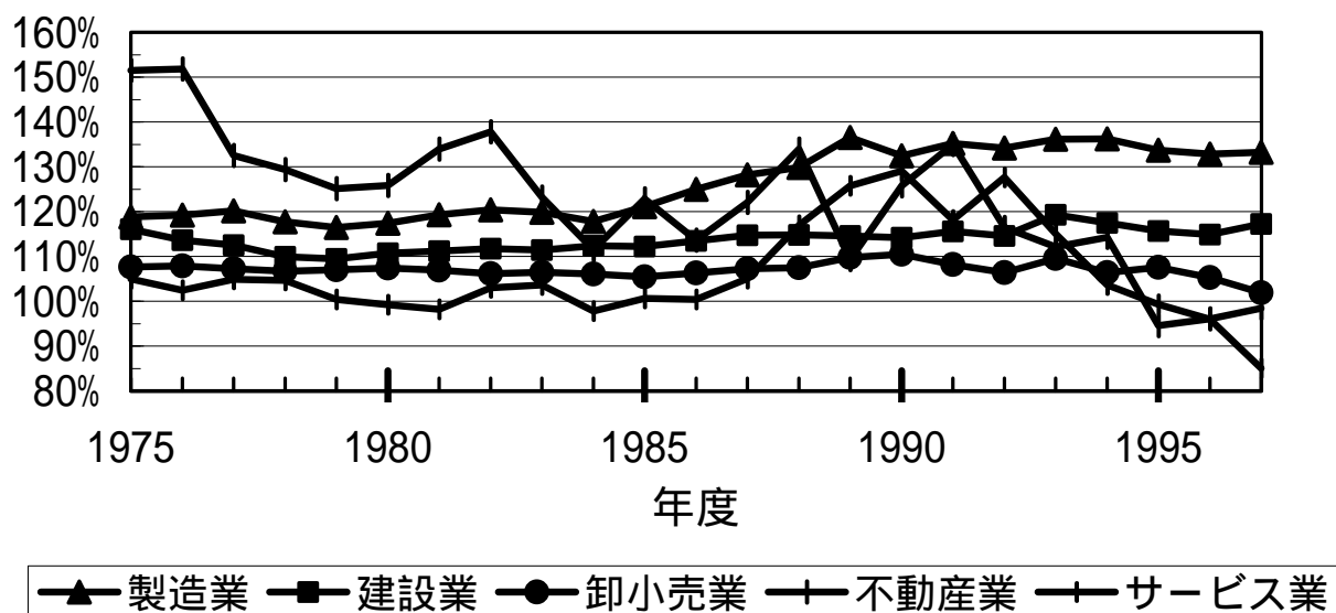
図 4 7 流動比率
